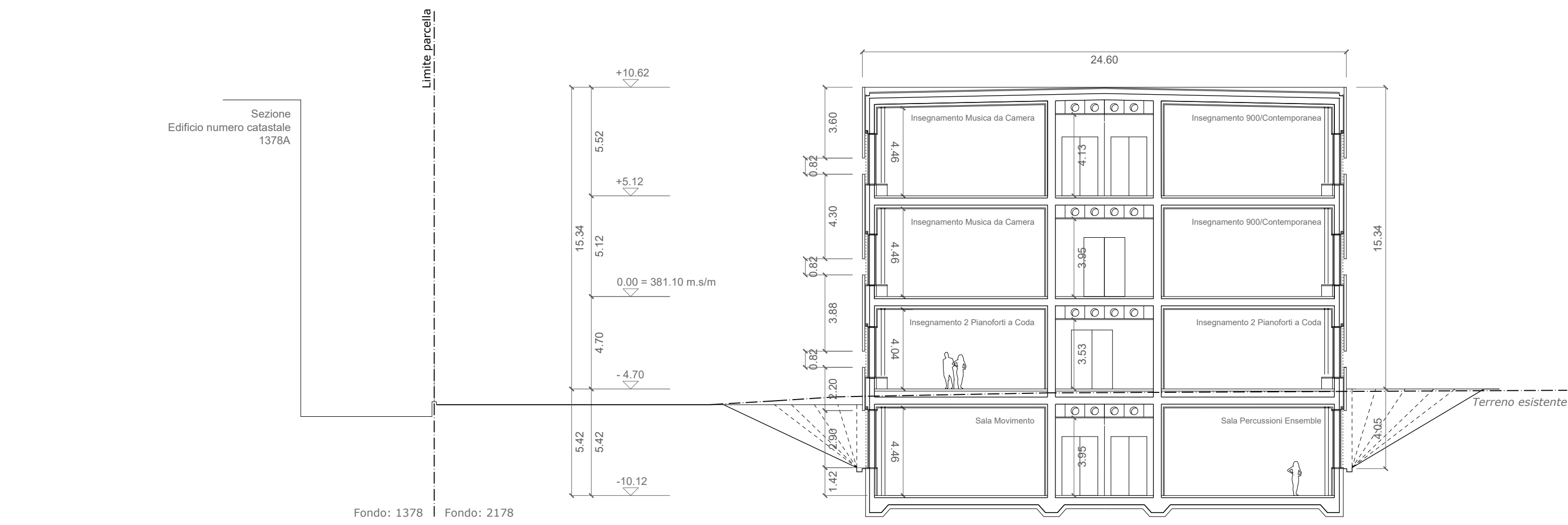
SEZIONE I - I
