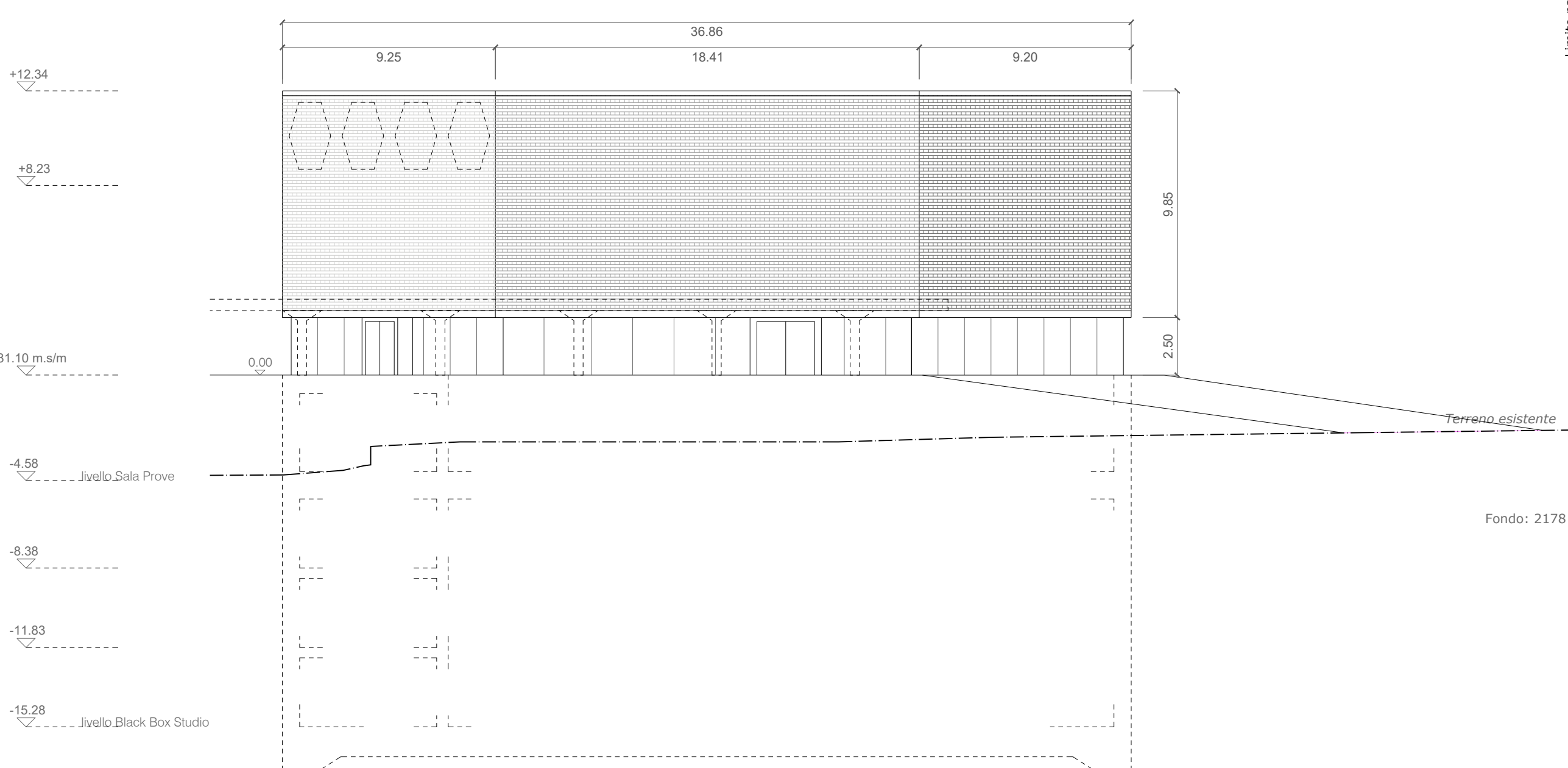
PROSPETTO EST (SALA CONCERTI / PROVE)
