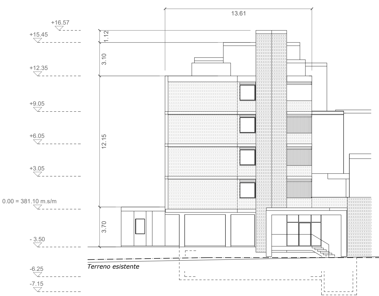
PROSPETTO SUD (STABILE A)
