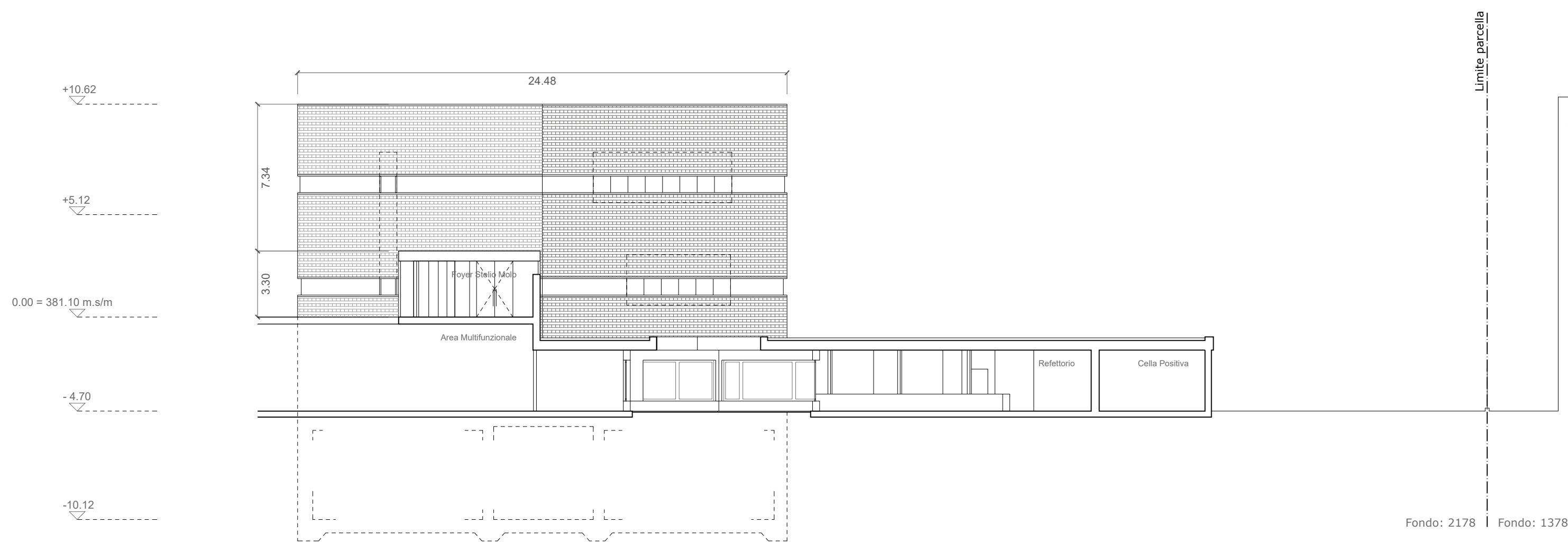
PROSPETTO OVEST (ALA DP2)
