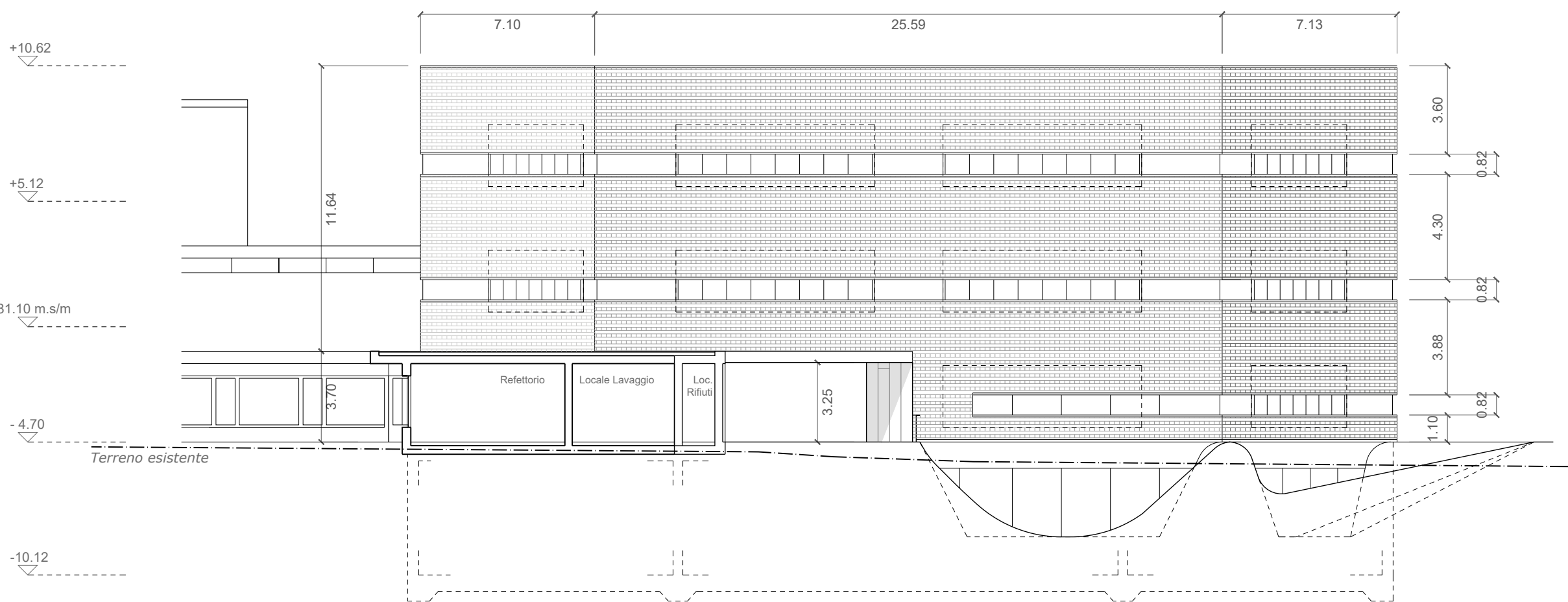
PROSPETTO SUD (ALA DP2)
