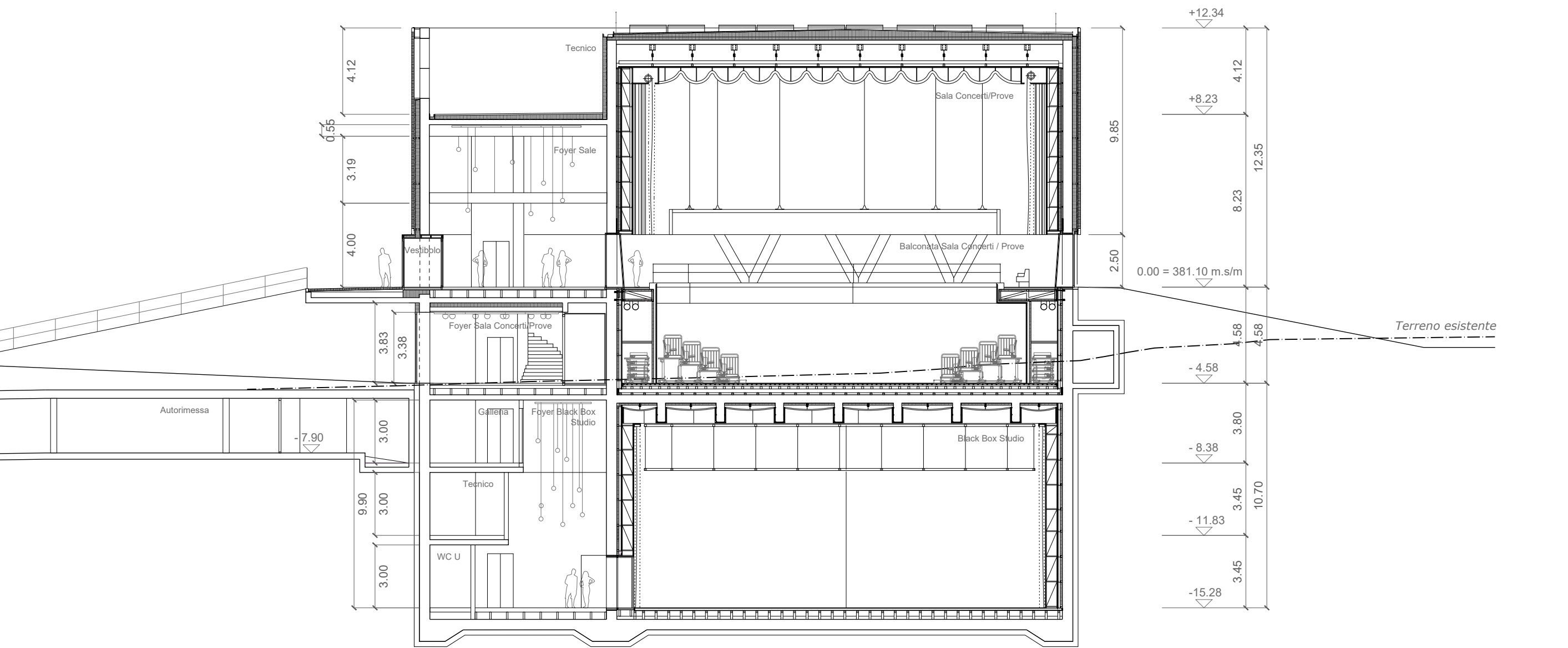
SEZIONE F - F
