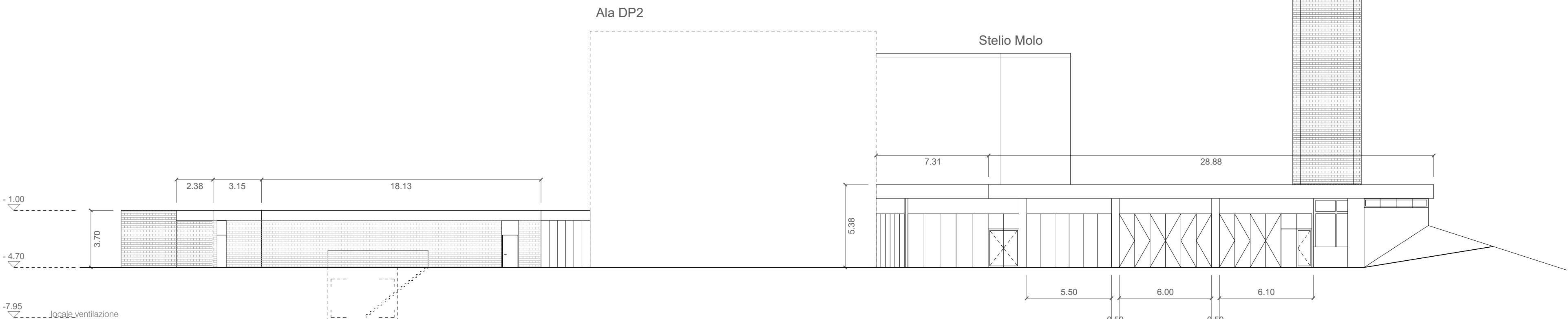
PROSPETTO EST CUCINA / ZONA CARICO - SCARICO (STABILE A)
