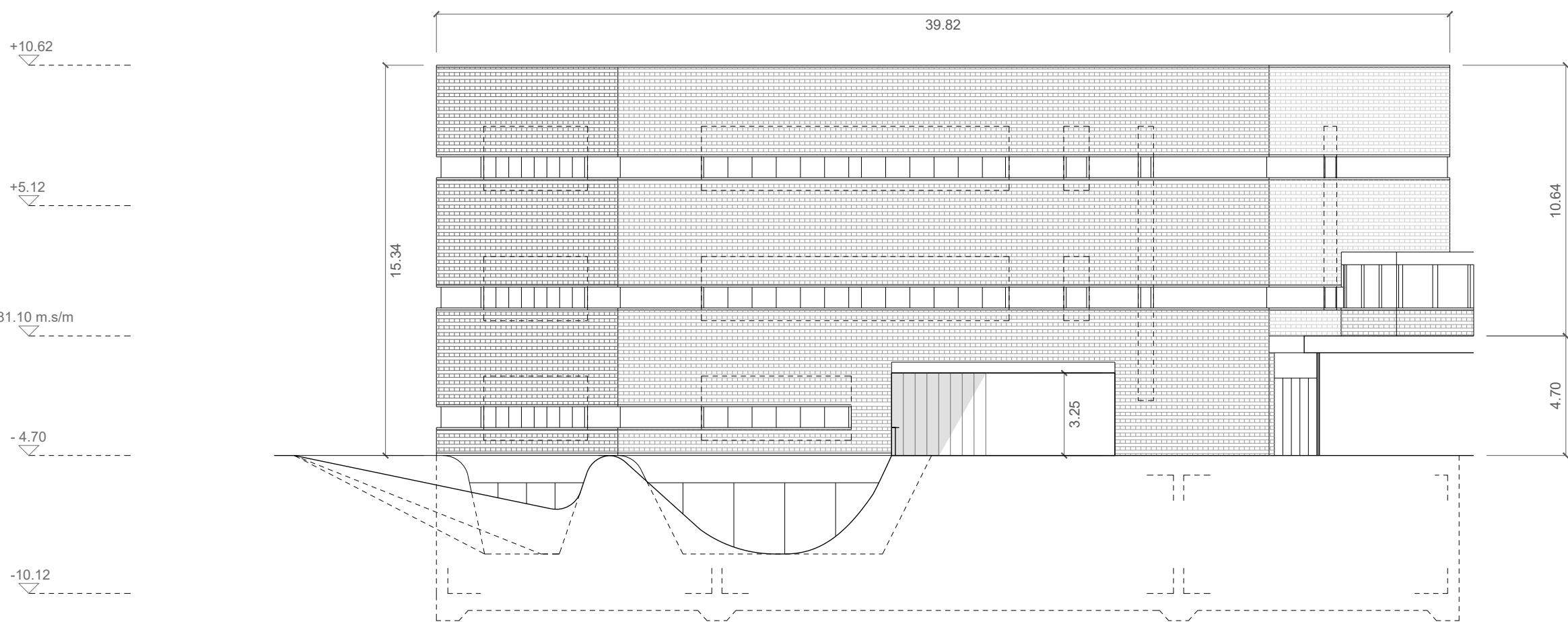
PROSPETTO NORD (ALA DP2)
