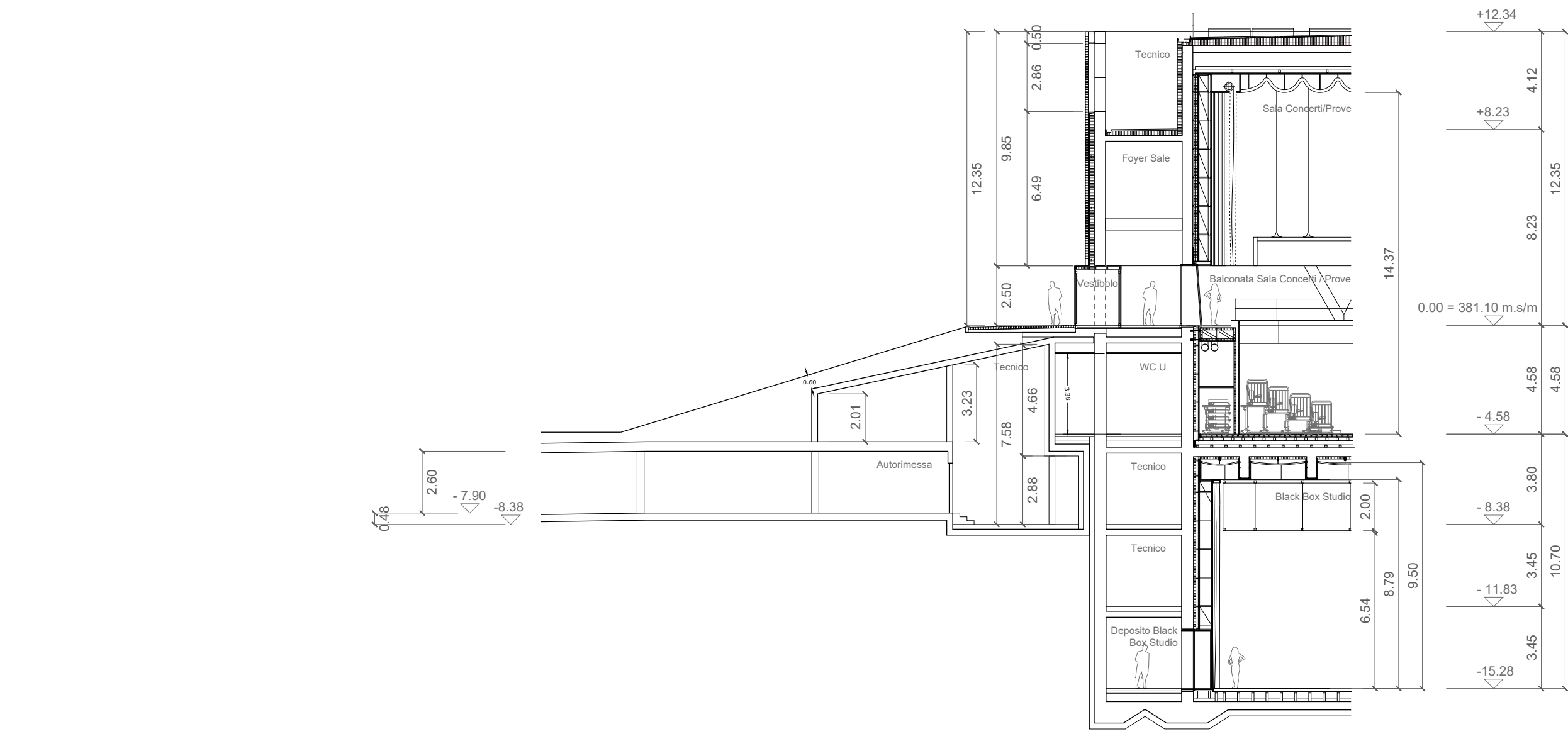
SEZIONE F' - F'
