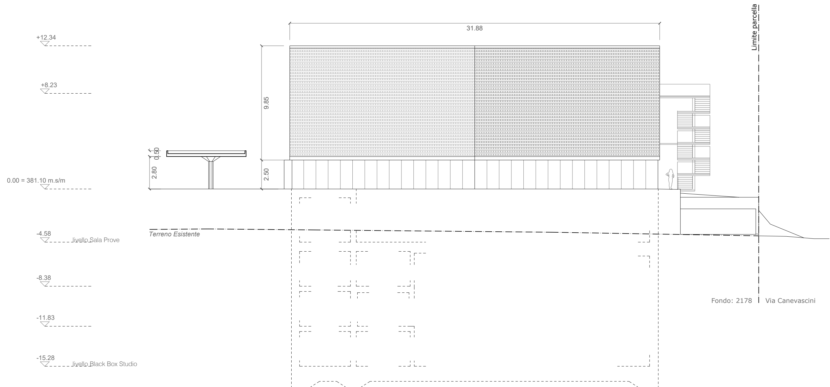
PROSPETTO NORD (SALA CONCERTI / PROVE)
