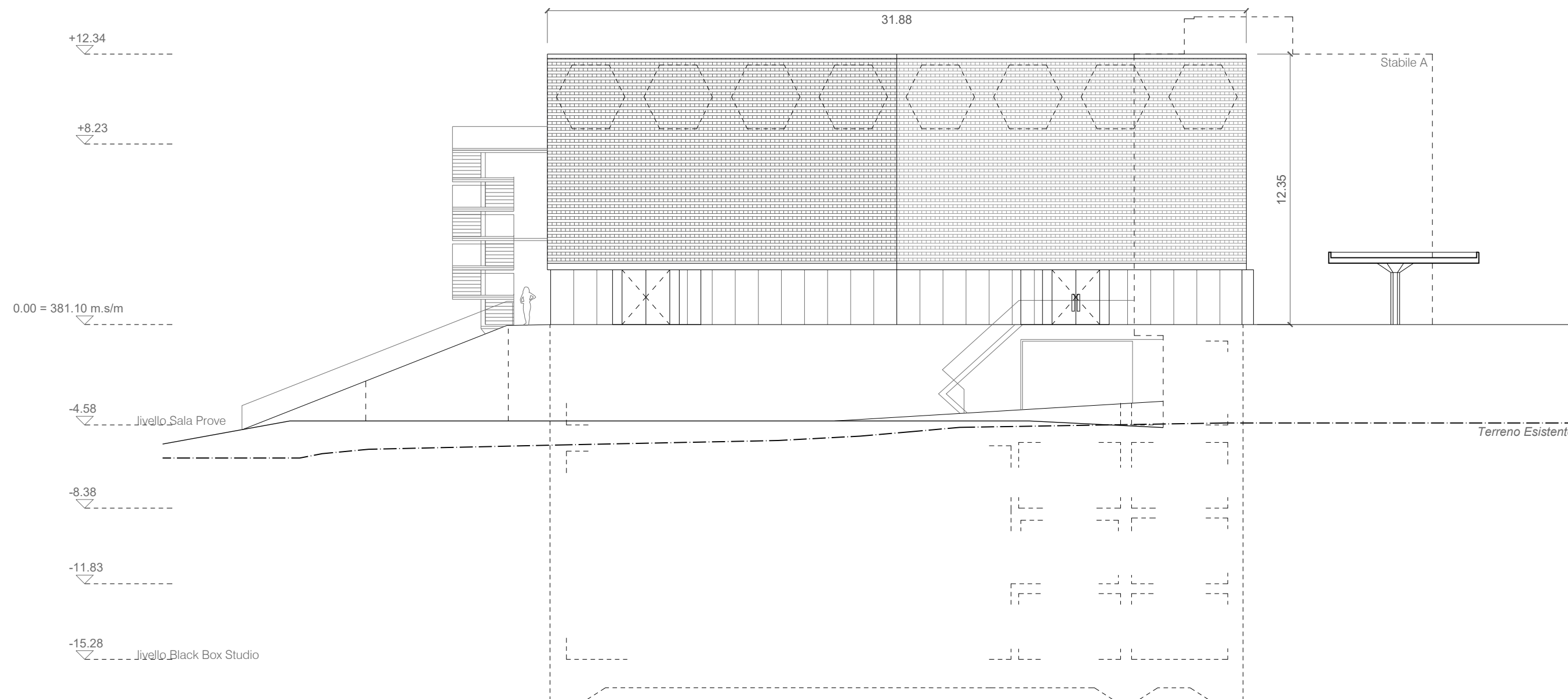
PROSPETTO SUD (SALA CONCERTI / PROVE)
